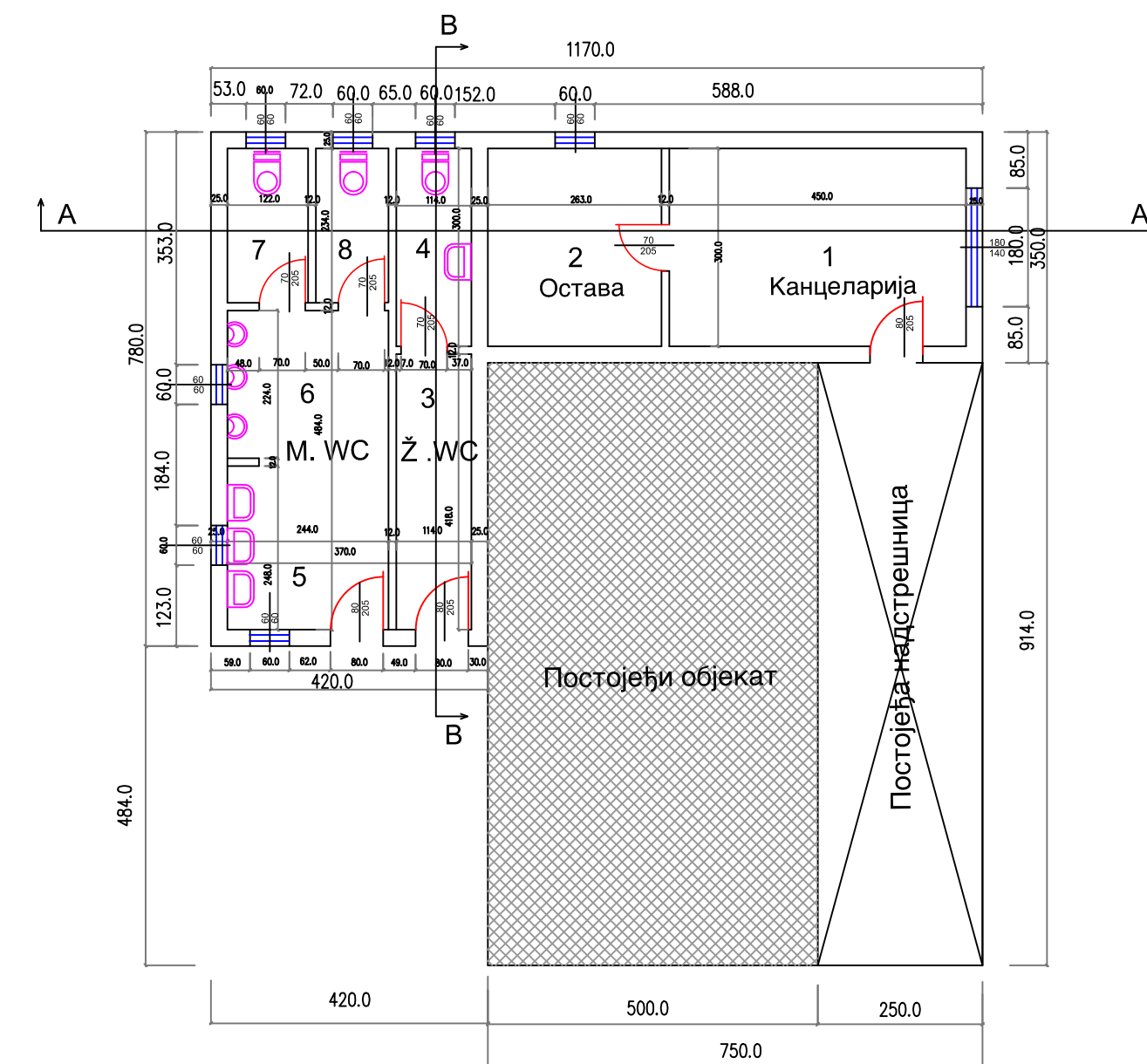
Основа приземља
