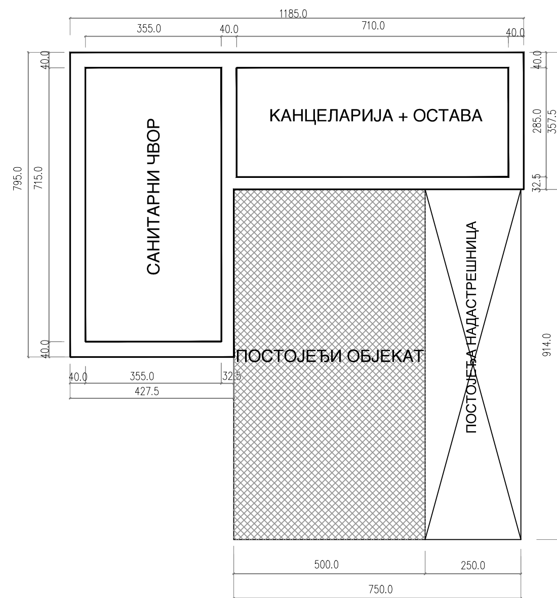
Основе темеља
